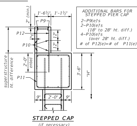
END ELEVATION
