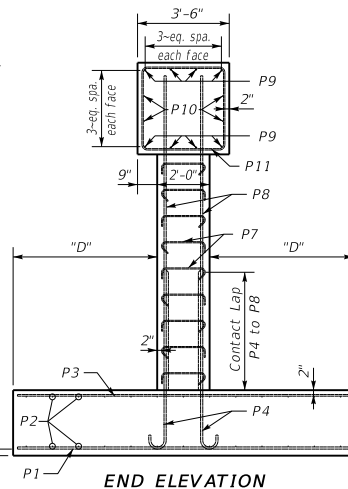
END ELEVATION
